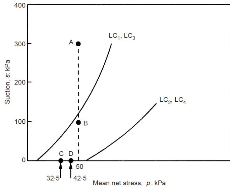
รูปที่ 3.1 ภาพร่างสถานะหน่วยแรงระหว่างเตรียมตัวอย่างดินเหนียวเกาหลีกับ LC curve ของแต่ชุดข้อมูล (Sivarkumar และ Wheeler, 2000)
