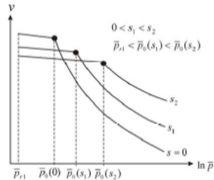
รูปที่ 1 ภาพร่างการคายออกของเส้นโค้งการอัดตัวปกติ
