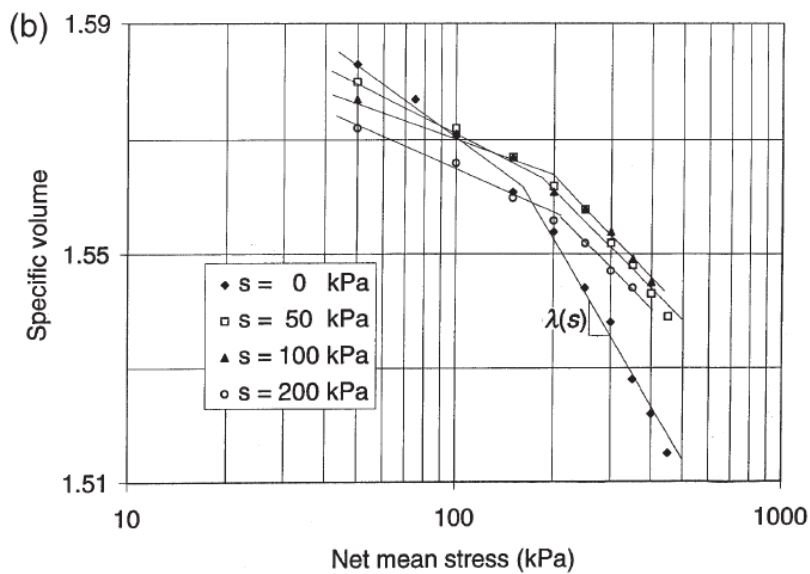
รูปที่ 4.22 เส้นการอัดตัวแบบไอโซโทรปิกของดินลมหอบสีเหลืองบดอัด (Chen et al., 1999)
