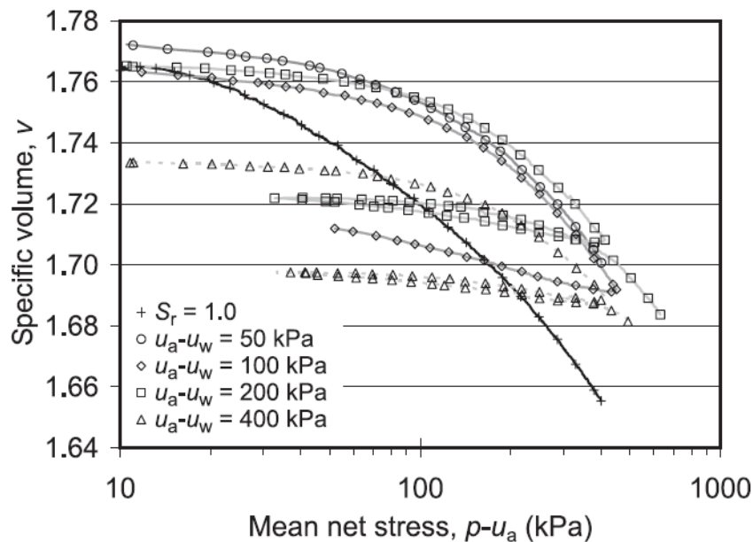
รูปที่ 3.9 เส้นโค้งการอัดตัวแบบไอโซโทรปิกของ Po silt บดอัด (Vassallo et al, 2007)
