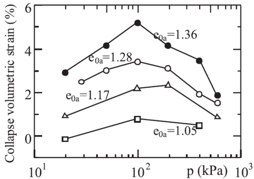
รูปที่ 4.26 ความสัมพันธ์ระหว่างหน่วยแรงสุทธิและความเครียดเชิงปริมาตร
