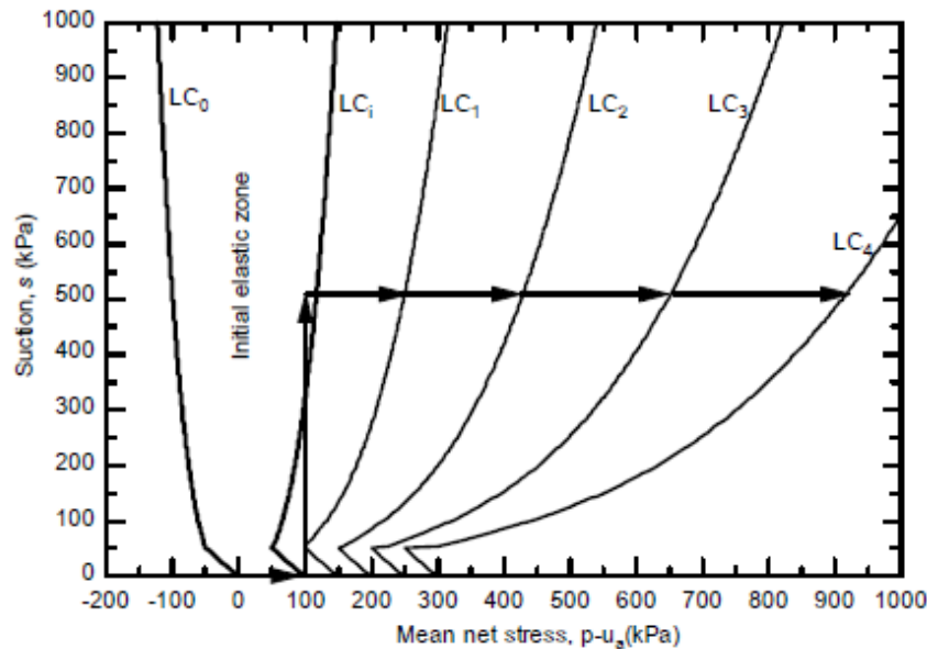
รูปที่ 3 LC curve ของดินเมื่ออัดตัวภายใต้สภาวะอิ่มตัวด้วยน้ำจาก 100 ไปยัง 150 200 250 และ 300 kPa ตามลำดับ
