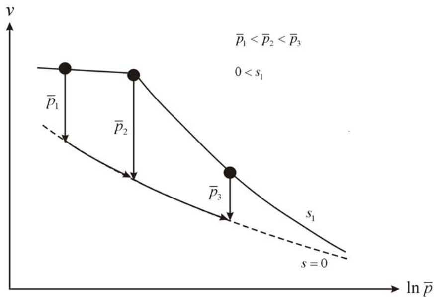
รูปที่ 3.19 ภาพร่างระดับการพังทลายภายใต้หน่วยแรงสุทธิต่าง ๆ บนระนาบ v - \ln \bar{p}
