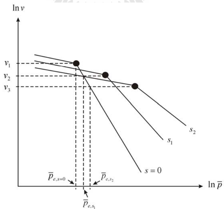
รูปที่ 4.9 หน่วยแรงสุทธิตามมุมบรรเทา \ln v - \ln \bar{p}
