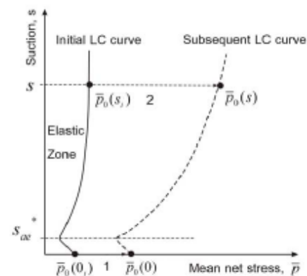
รูปที่ 2 ภาพร่าง LC curve ของการเพิ่มหน่วยแรงสุทธิ
