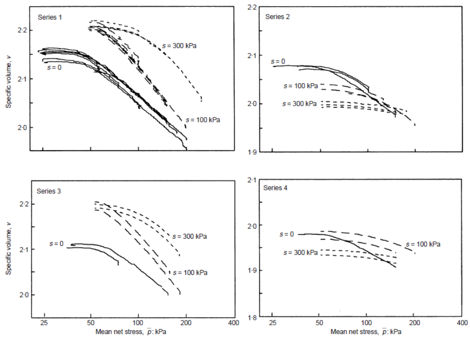
รูปที่ 3.2 เส้นโค้งการอัดตัวแบบไอโซโทรปิกของดินเหนียวเกาหลีชนิดอัด (Sivarkumar and Wheeler, 2000)
