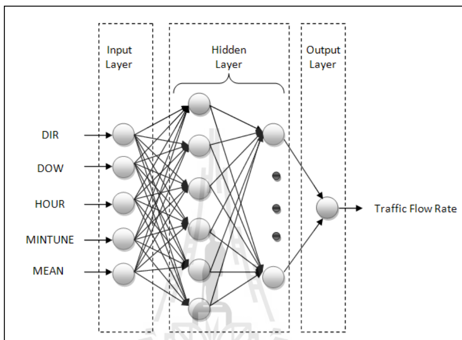
รูปที่ 3.38 โครงสร้างของเครือข่ายประสาทเทียมสำหรับการสร้างแบบจำลองการจราจร
