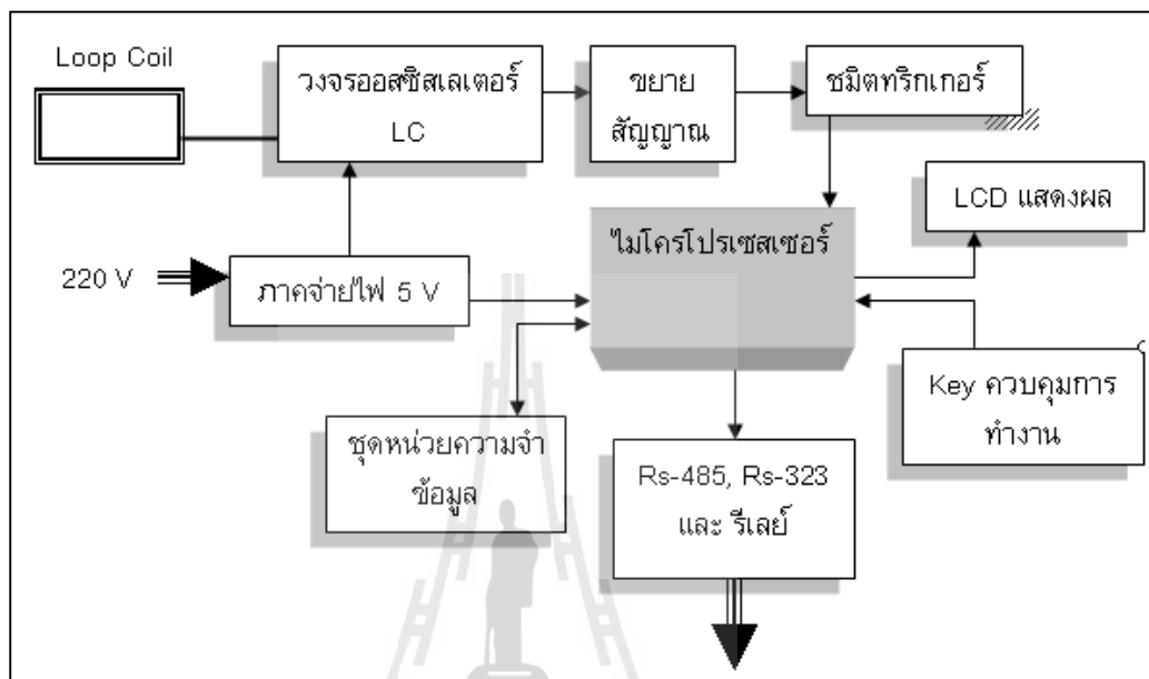
รูปที่ 2.9 ลักษณะวงจรพื้นฐานของส่วนเครื่องตรวจจับยานพาหนะแบบลู่วิ่ง
