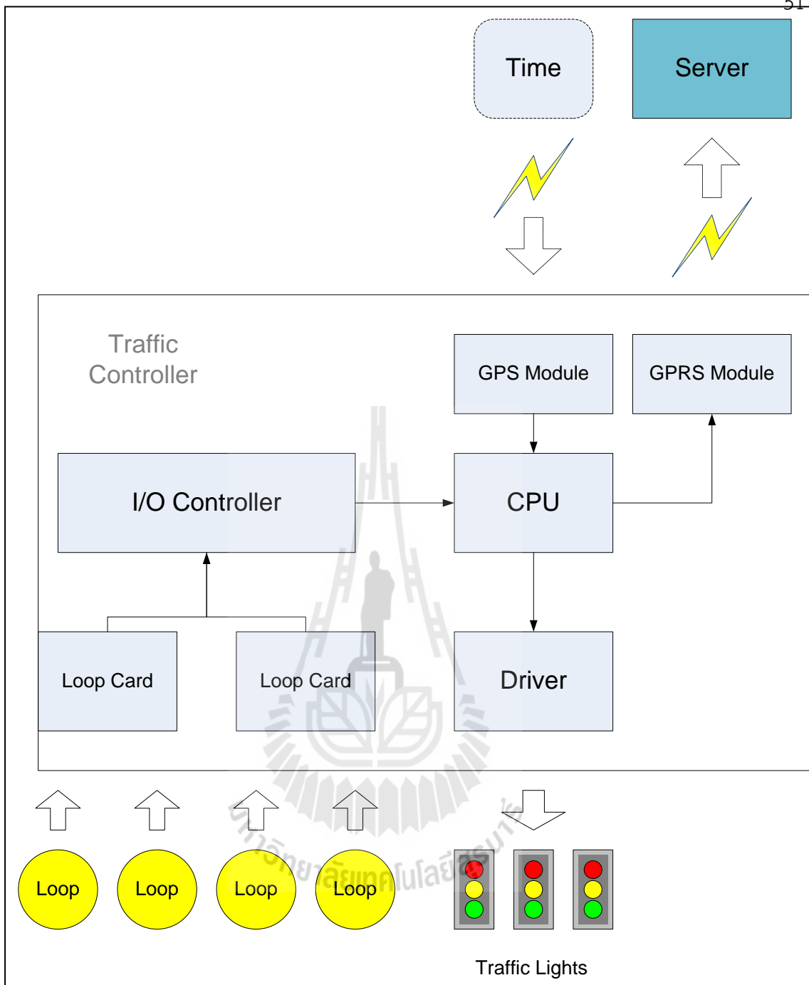
รูปที่ 3.35 ลักษณะการทำงานของระบบสัญญาณไฟจราจร
