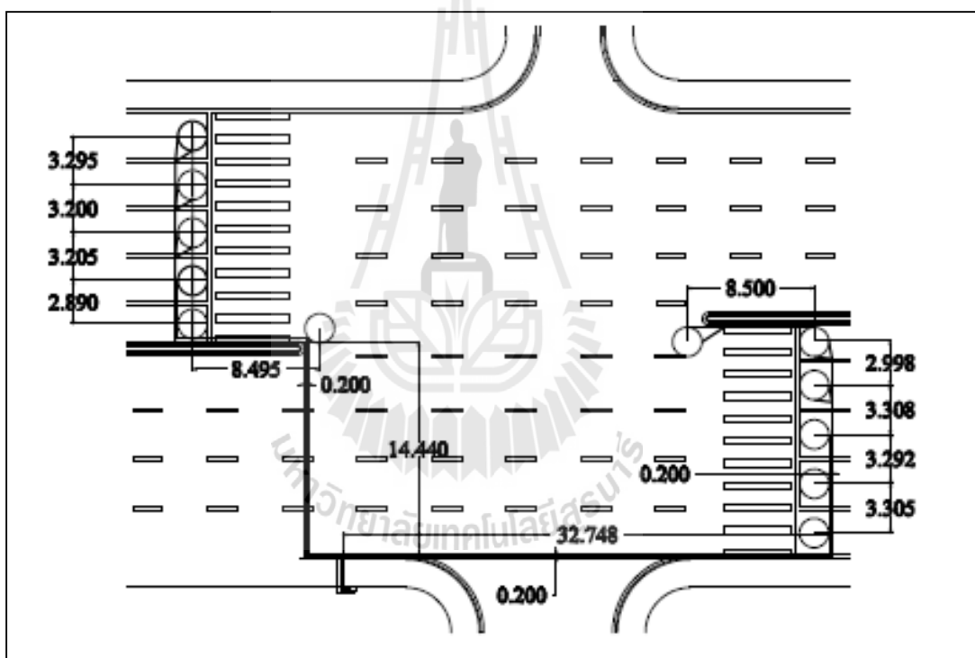
รูปที่ 3.6 แสดงการวางตำแหน่ง Loop Detector ที่แยกสำโรงจันท์
