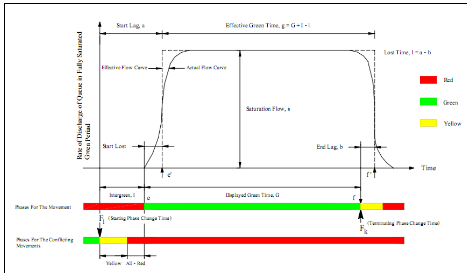
รูปที่ 2.4 แบบจำลองปริมาณการจราจรอิมตัวและไฟเขียวประสิทธิภาพของ Akcelik [ที่มา: Akcelik (1981)]
