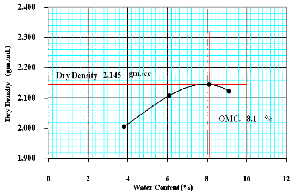
รูปที่ 4.7 ความสัมพันธ์ปริมาณน้ำกับความหนาแน่นของวัสดุพื้นทางเดิม
